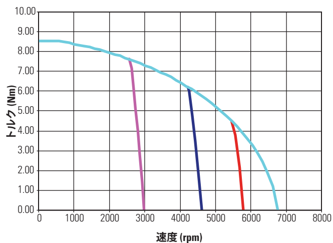
KBM(S)-25X02 連続トルク
