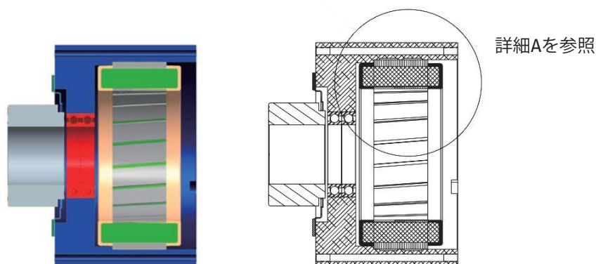
2D表示
