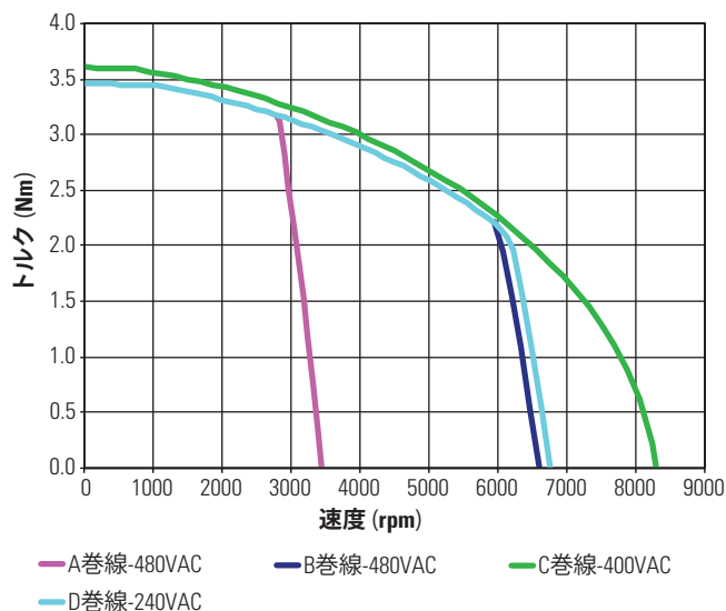
KBM(S)-17X02 連続トルク
