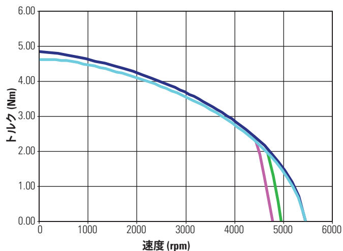
KBM(S)-25X01 連続トルク
