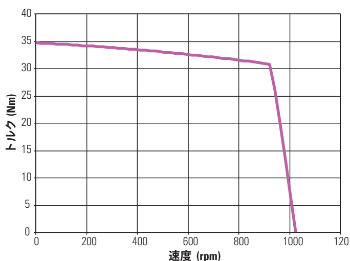
KBM(S)-43X04 連続トルク
