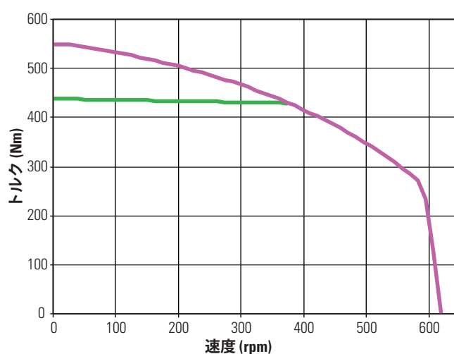
KBM(S)-118X03 連続トルク
