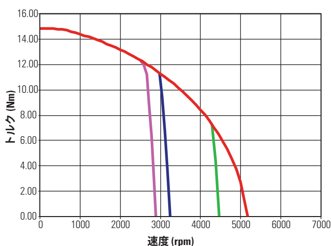
KBM(S)-25X04 連続トルク
