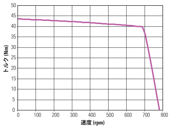
KBM(S)-43X05 連続トルク
