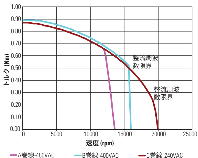
KBM(S)-10X02 連続トルク
