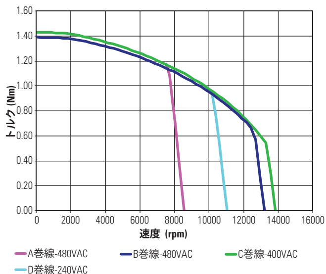
KBM(S)-10X04 連続トルク
