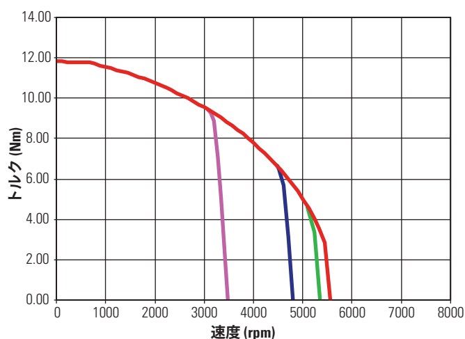
KBM(S)-25X03 連続トルク
