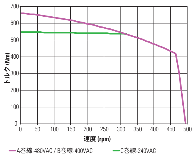
KBM(S)-118X04 連続トルク
