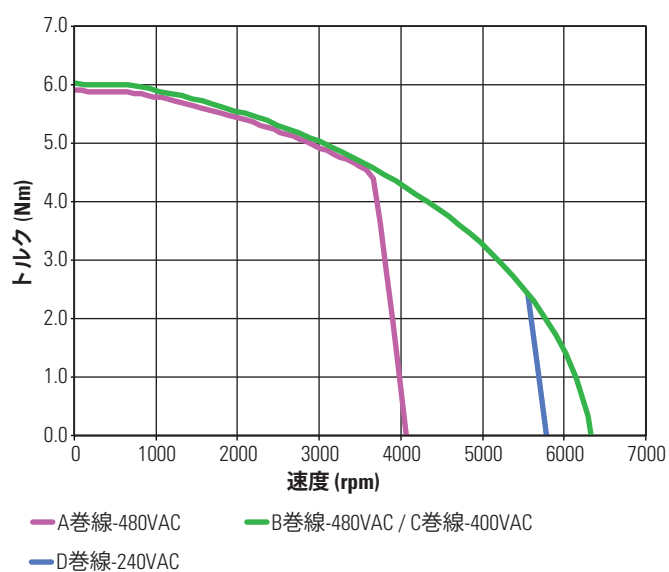
KBM(S)-17X04 連続トルク
