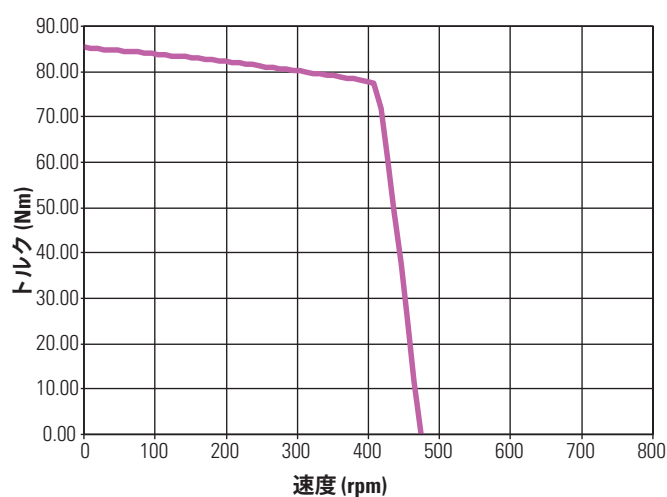
KBM(S)-57X04 連続トルク
