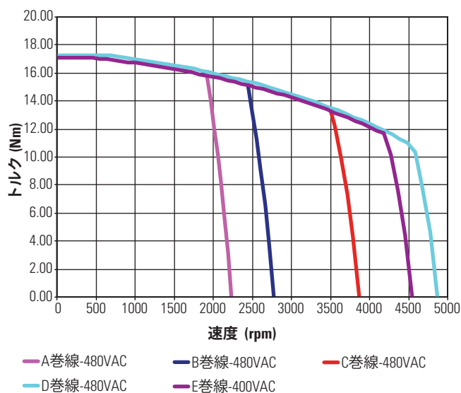
KBM(S)-35X02 連続トルク
