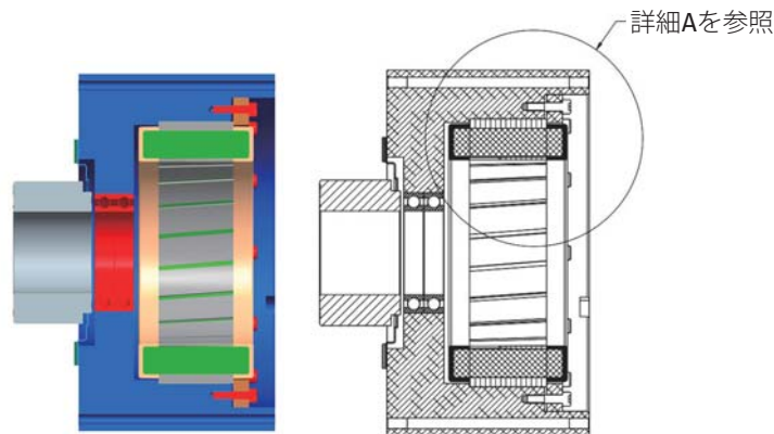
2D表示
