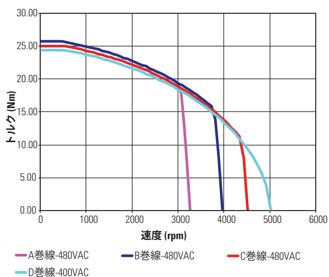
KBM(S)-35X04 連続トルク
