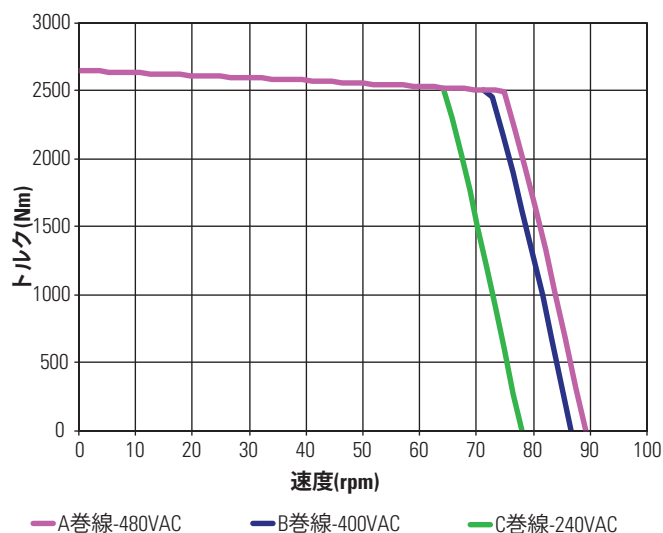
KBM(S)-260X02 連続トルク
