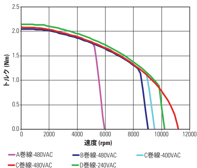
KBM(S)-14X02 連続トルク
