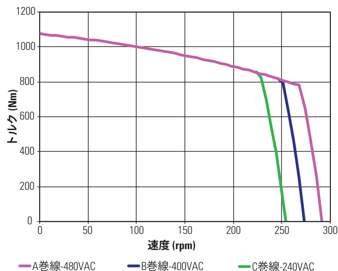
KBM(S)-163X02 連続トルク
