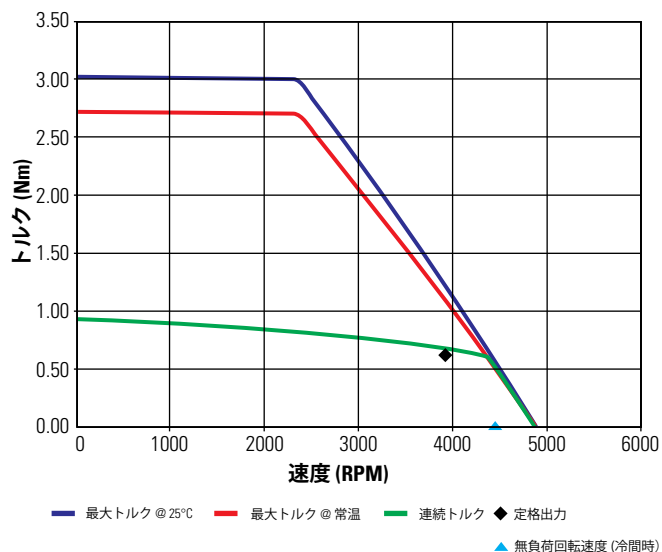
TBM(S)-7615-A 48Vdc (6 step で計測)
